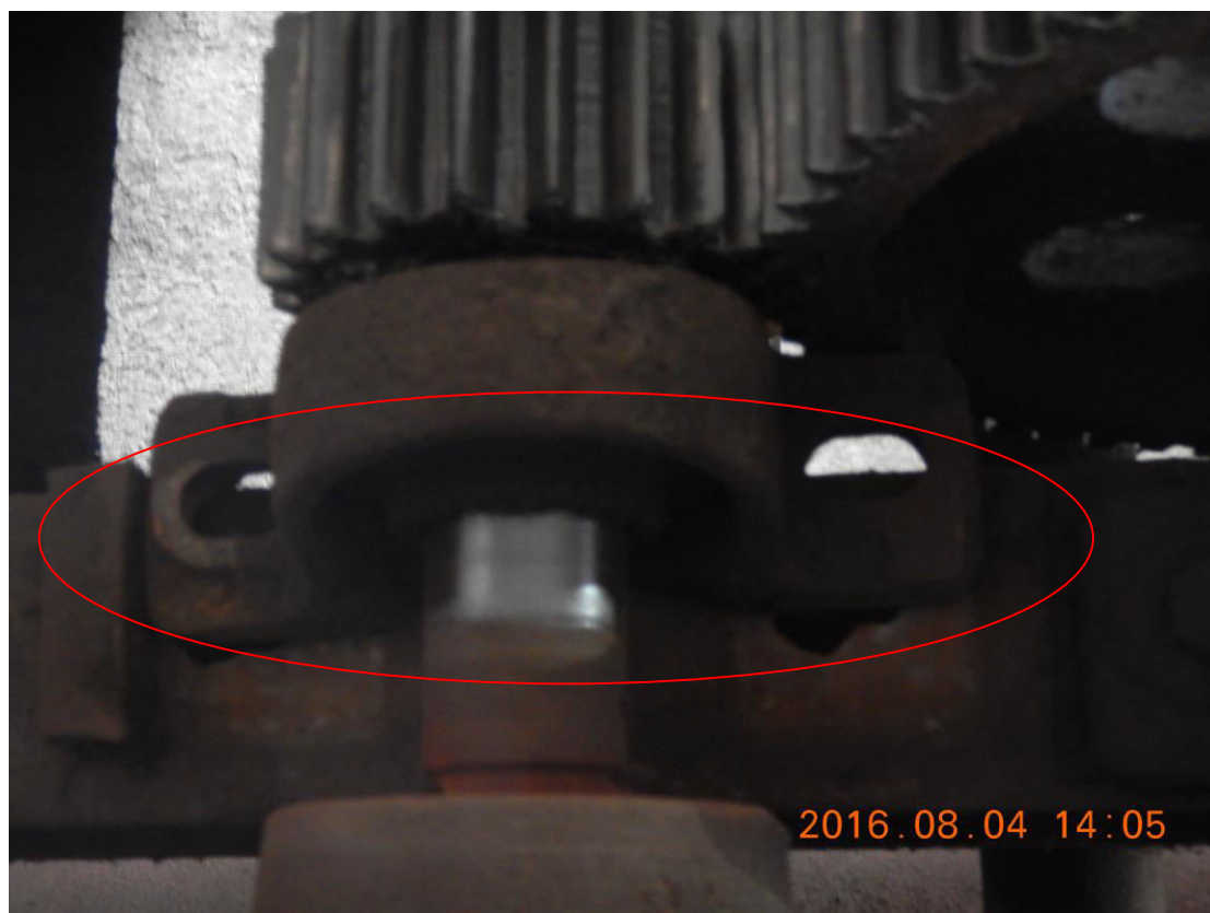
橫行馬達傳動軸軸承座鬆脫
